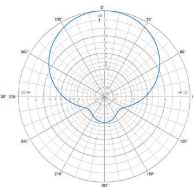
H-Plane | 155 MHz
