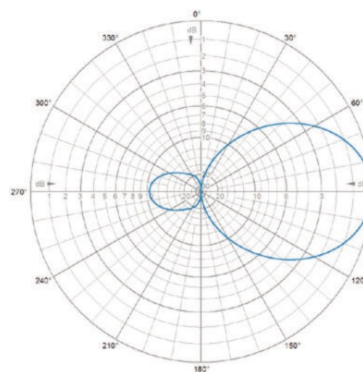
E-Plane | 155 MHz
