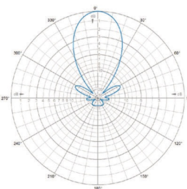
H-Plane | 445 MHz
