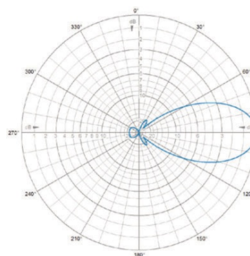
E-Plane | 445 MHz
